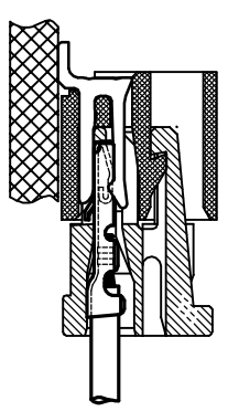
嵌合状态
