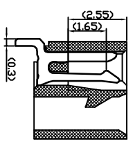
剖面 A-A
